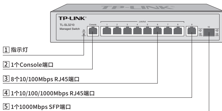
图1-16 TL-SL3210前面板示意图
