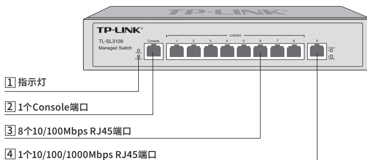
图1-17 TL-SL3109前面板示意图
