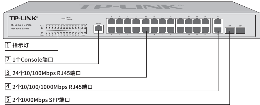
图1-12 TL-SL3226-Combo前面板示意图
